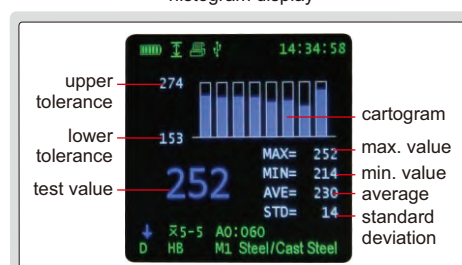
histogram display
